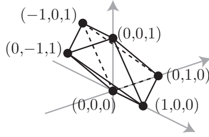
図 21: Q^{1,1,1} のトーリック図形
