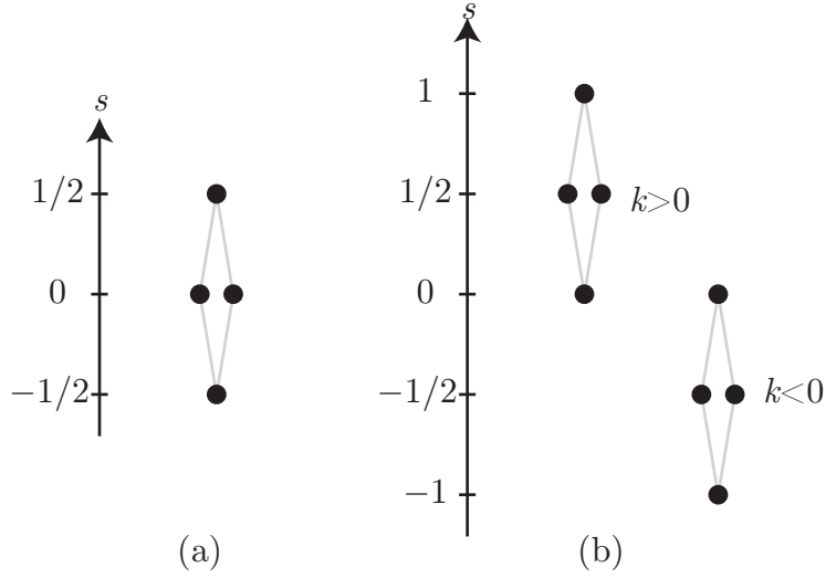
図 1: (a) 有質量カイラル多重項に含まれる粒子のスピンの分布 (b) 有質量ベクトル多重項に含まれる粒子のスピンの分布
