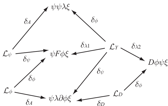
図 19.3: ゲージ場に結合したハイパー多重項の作用の超対称変換による変分の相殺。ここでは重力は無視し、パラメータ空間は平坦であると仮定しているが、フェルミオンについて高次の項は全て考慮されている。
