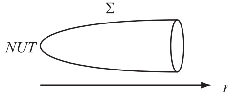
図 15.5: D6-ブレーンに端を持つ開弦は、11 次元超重力理論においては Taub-NUT 空間の非コンパクト 2-サイクルに巻きついた M2-ブレーンとして表される。
