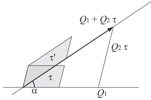
図 15.4: プレーンの電荷を Q^2 = 0 に取るための SL(2, \mathbf{Z}) 変換の Z -平面上での様子
