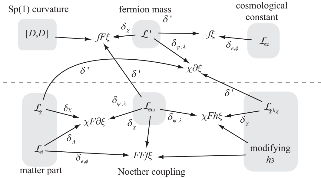
図 19.4: 重力に結合した 6 次元ベクトル多重項の作用の超対称変換による変分の相殺の様子。破線より上の部分はゲージ群が \text{Sp}(1)_R を含む場合にのみ必要である。
