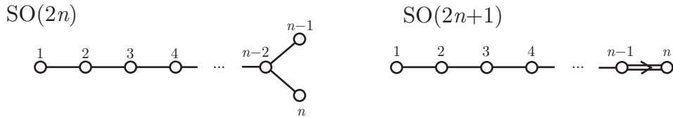
図 1.1: SO(2n) および SO(2n+1) のディンキン図形
