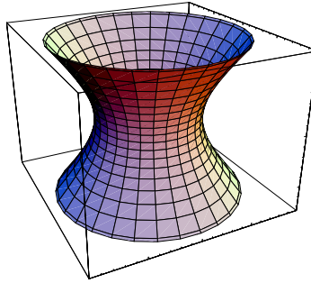
図 13.4: \text{AdS}_2 上にとった大域的座標。図中の縦の線が t が一定、横の線が r が一定の線を表している。この図では時間方向が循環しているように見えるが、実際には被覆として定義される。(adscoordinate.nb)
